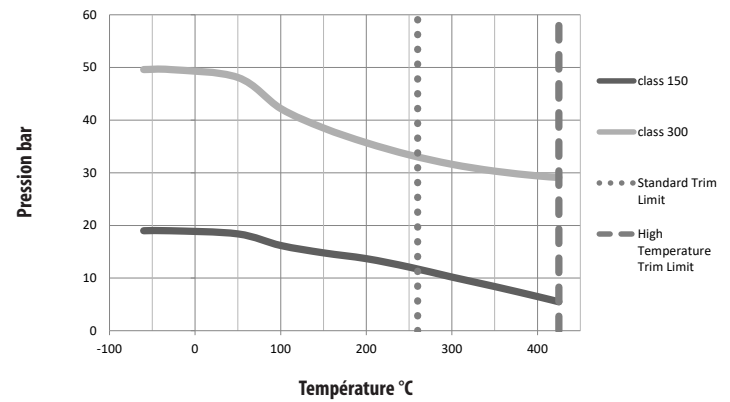
Pression et température ASTM A351 Gr. CF8M
