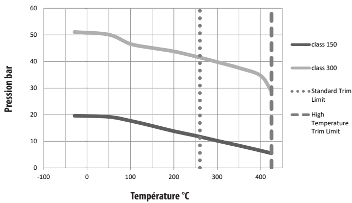
Pression et température ASTM A216 Gr. WCB
