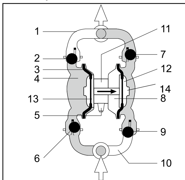
Рис. 2: Конструкция насоса
