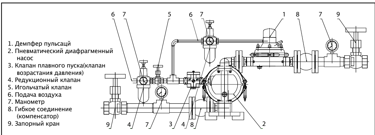
Чертёж 2
