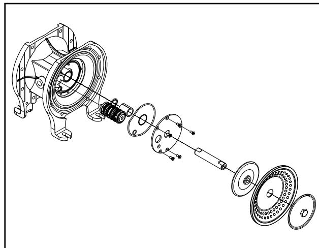
Рис. 22: Насос ДН с внутренним распределительным клапаном
