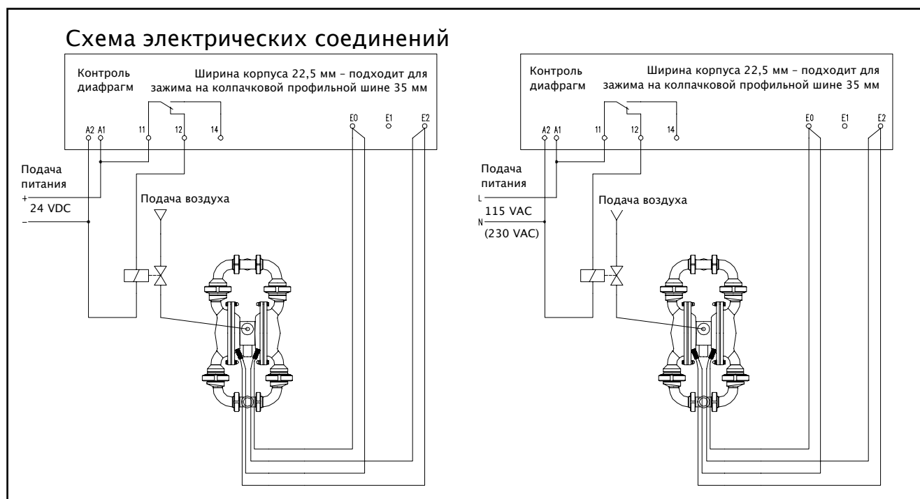
Рис. 6: Схема электрических соединений датчиков утечек
