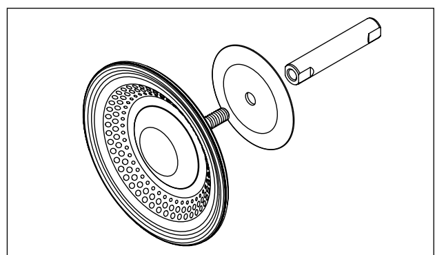
Рис. 14: Монтаж диафрагмы porpedE4®.
