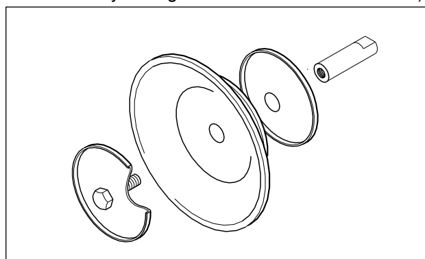
Obr. 13: Montáž membrán s vnitřním a vnějším talířem
