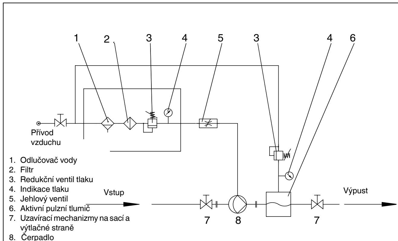
obr. 4: Příklad instalace čerpadla
