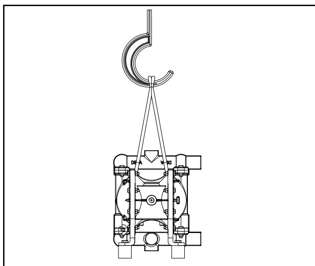
obr. 1: Přeprava čerpadla
