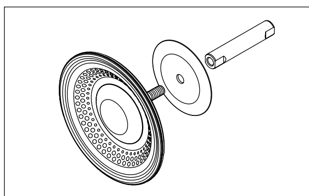
obr. 14: Montáž membrány noppedE4®
